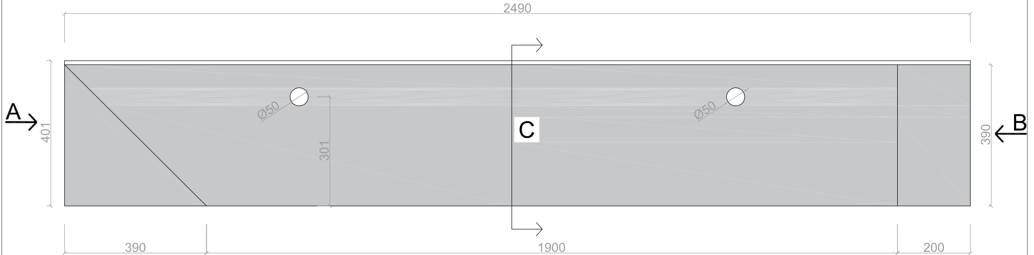
ALZADO FRONTAL. GEOMETRÍA
