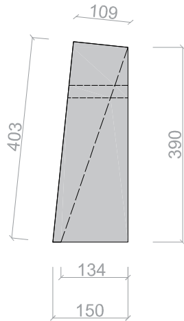
VISTA A
