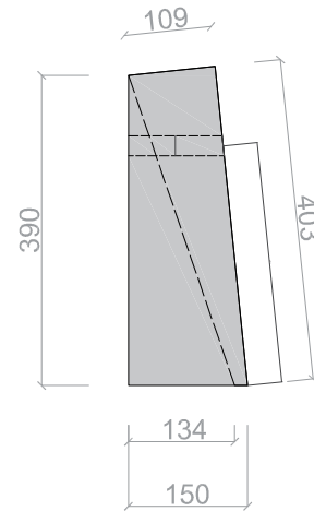
VISTA B
