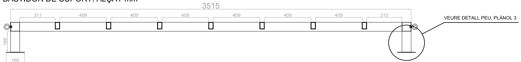
BASTIDOR DE SUPORT. ALÇAT mm
